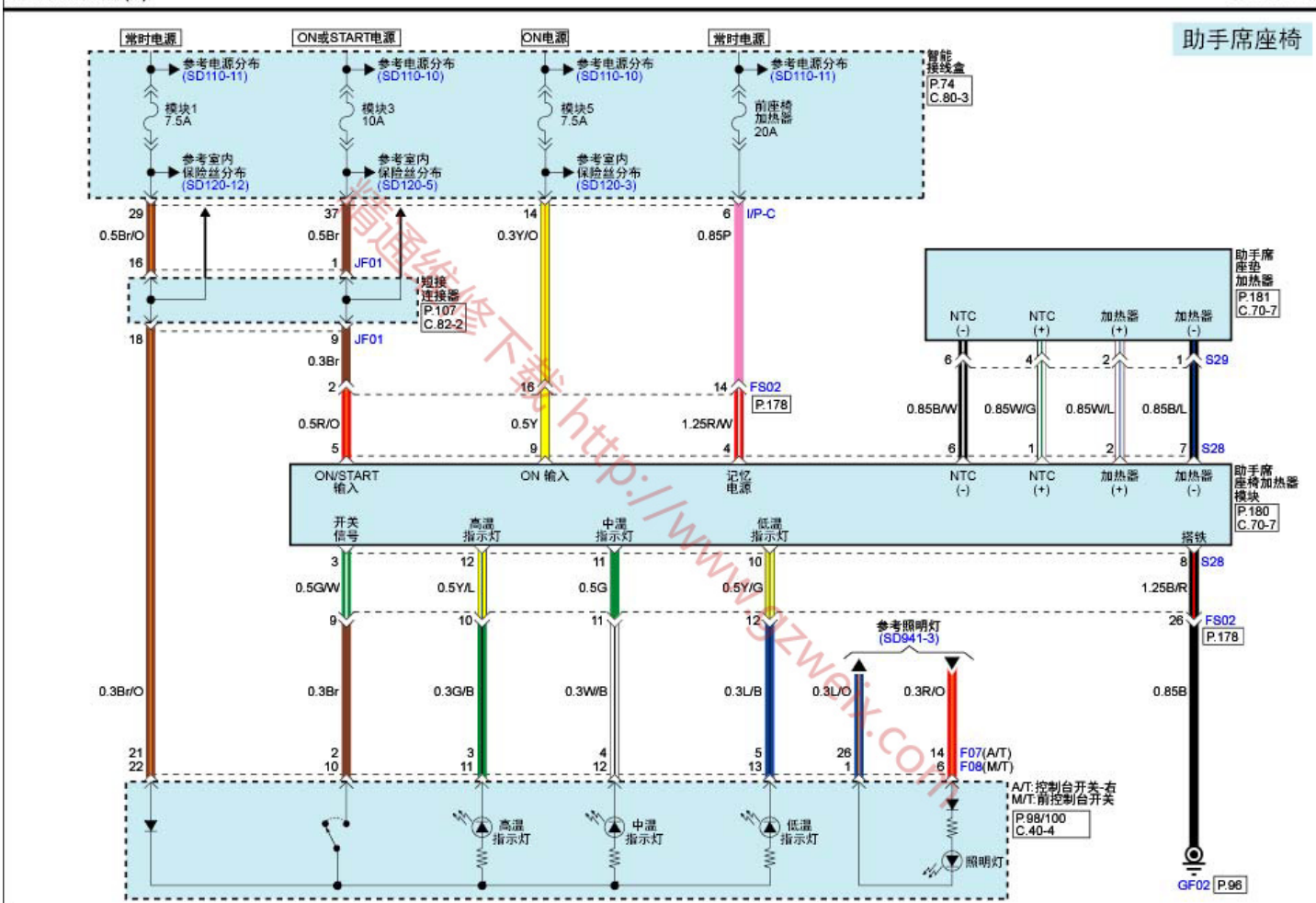
座椅加热器(2)
